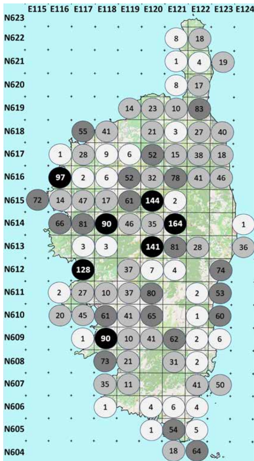
Figure 3.- Carte des prospections, bilan 2018 en nombre d'espèces répertoriées.
