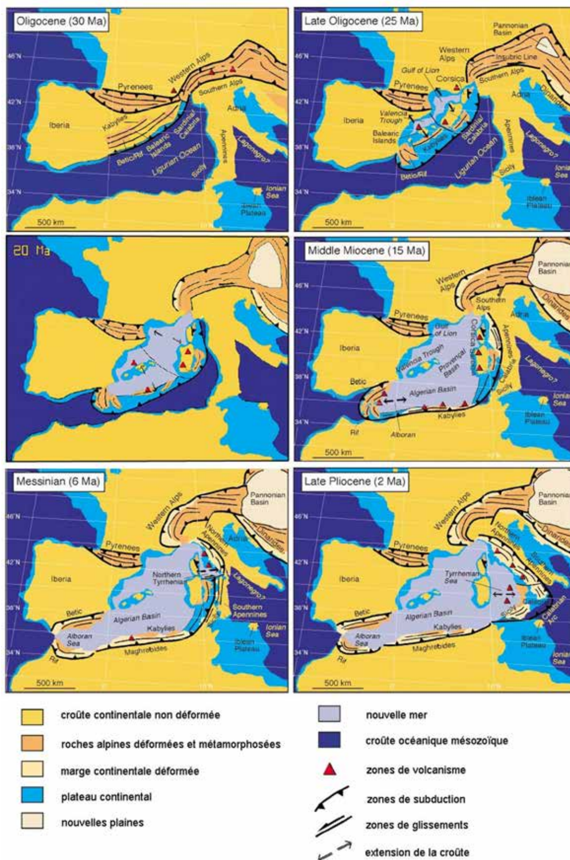
Figure 4.- Dérive géographique des îles de la Méditerranée occidentale depuis l'Oligocène (d'après ROSENBAUM et al. in DE CHECA, 2015).
