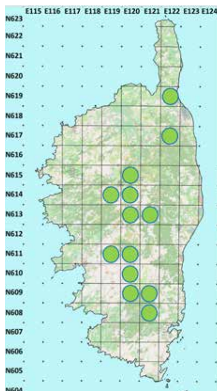
Palliduphantes gladiola , Hautes-Alpes, Corse
